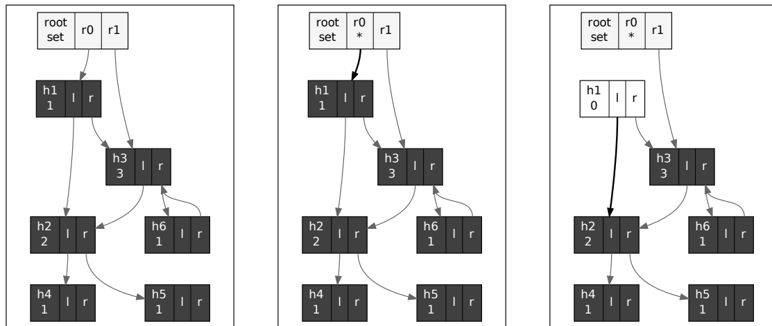
(a) Estado inicial del grafo de conectividad. (b) Al ejecutarse update(r0, null) , se comienza por visitar la celda h1 . (c) Se decrementa el contador de h1 quedando en 0 (pasa a ser basura ). Se elimina primero h1.l y luego h1.r .
