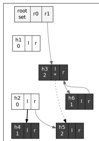
(c) Se decreenta el contador de h2 y queda en 0 (pasa a ser basura ). Se eliminan las referencias a las hijas.
