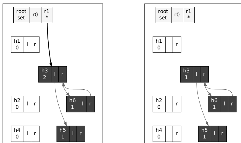
(a) El ejecutarse update(r1, null) se visita la celda h3 . (b) Se decrementa el contador de h3 pero sigue siendo mayor que 0 por el ciclo.
