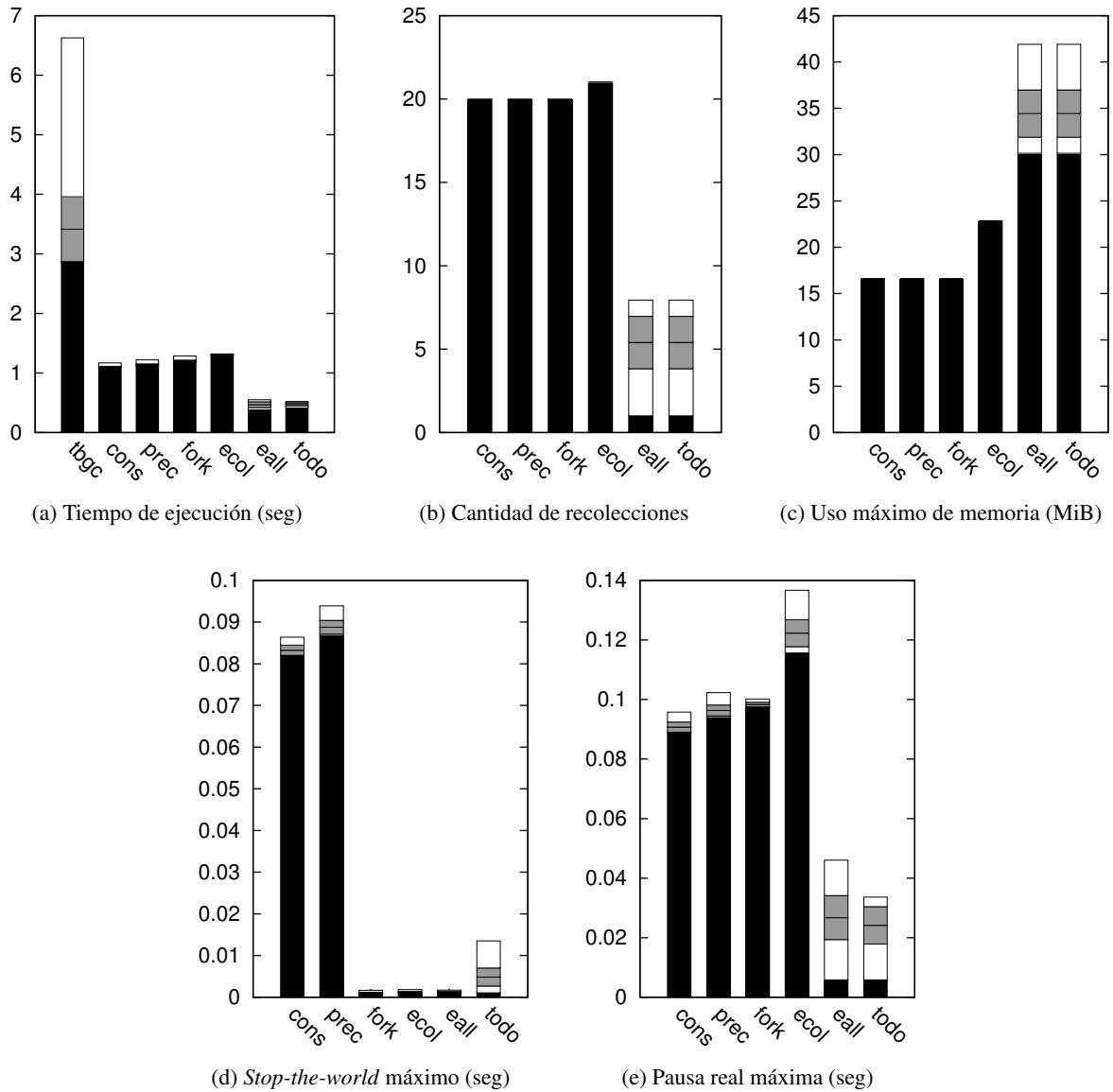
Figura 5.18: Resultados para voronoi (utilizando 1 procesador). Se presenta el mínimo (en negro), la media centrada entre dos desvíos estándar (en gris), y el máximo (en blanco) calculados sobre 50 corridas (para tiempo de ejecución) o 20 corridas (para el resto).
