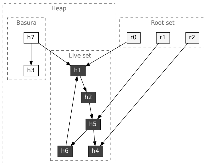
Figura 3.1: Distintas partes de la memoria, incluyendo relación entre basura , live set , heap y root set .
